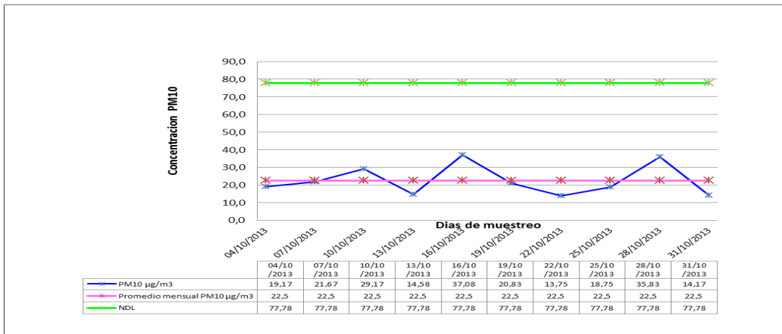
Concentración de PM10 Vs Norma diaria de Calidad del Aire mes de octubre de 2013
