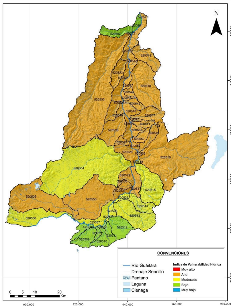
Figura 21 Distribución espacial del IVH, para las subcuencas de la cuenca hidrográfica del Río Guátara.
