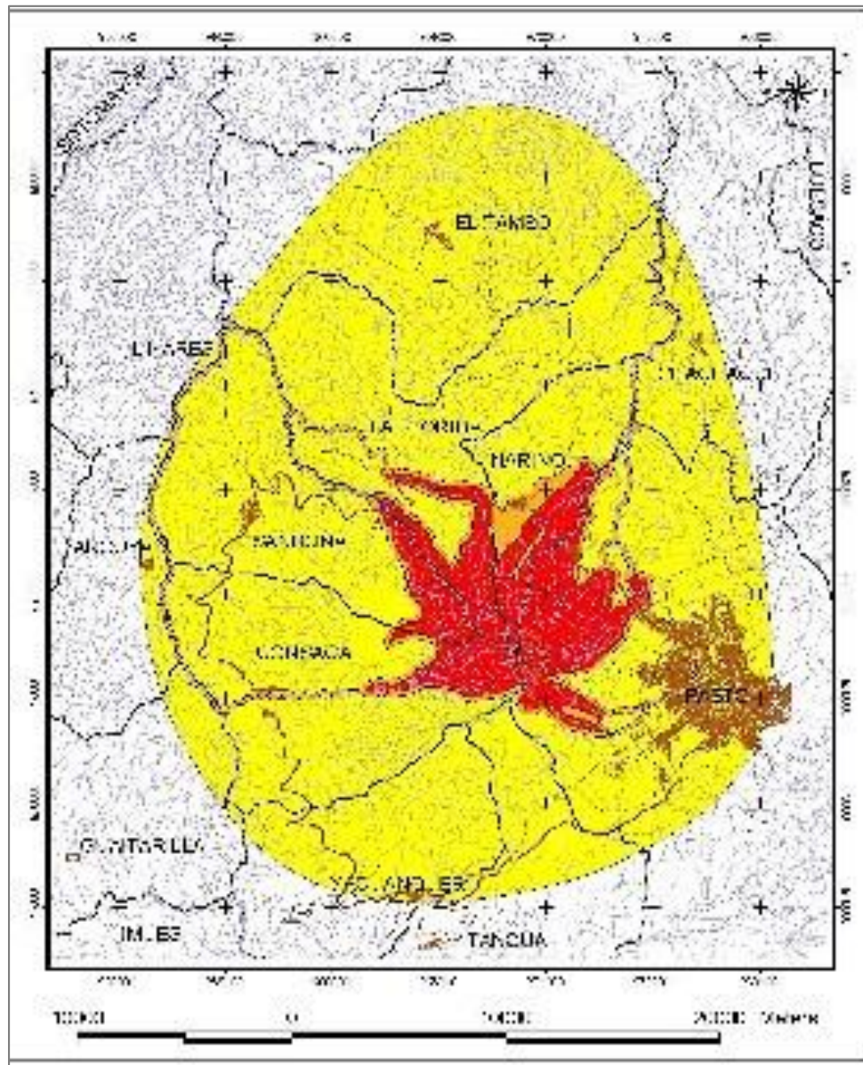
Figura 30 Mapa de amenaza volcánica del volcán Galeras
